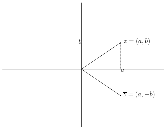
Figura 2.1: il piano di Argand–Gauss
