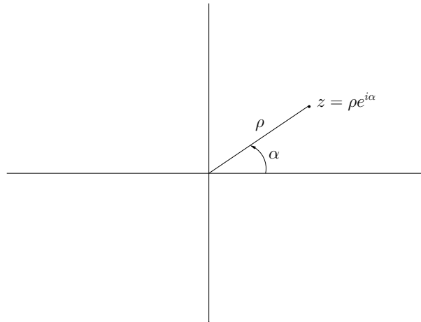
Figura 2.3: forma trigonometrica
